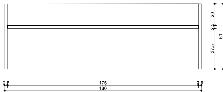
HORIZONTALNI PRESJEK
