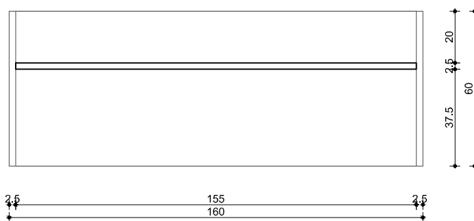
HORIZONTALNI PRESJEK
