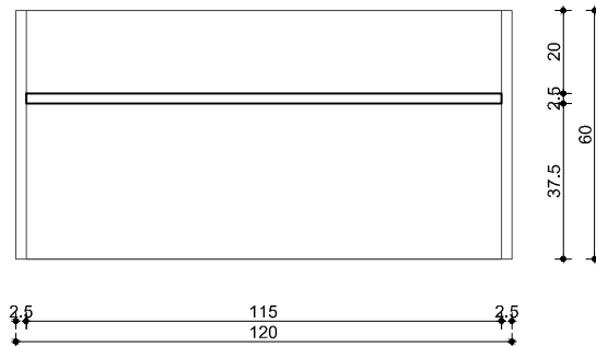
HORIZONTALNI PRESJEK
