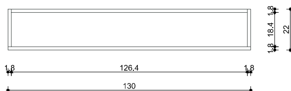
PRESJEK 1-1
