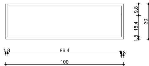
PRESJEK 1-1
