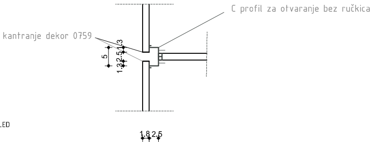
DETALJ OTVARANJA LADICE BEZ RUČKICA MJ 1:10
