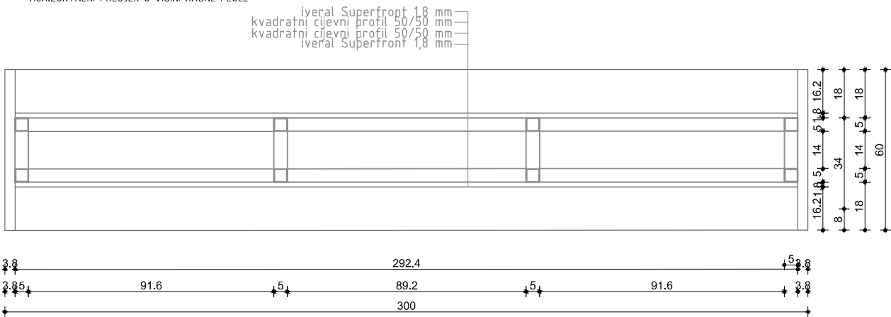
HORIZONTALNI PRESJEK U VISINI RADNE PLOČE
