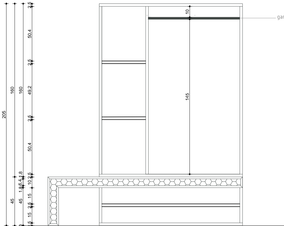
PRESJEK B-B
