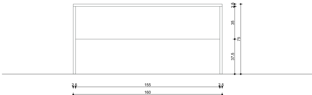
PRESJEK 1-1
