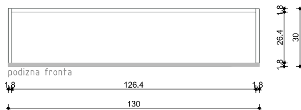
HORIZONTALNI PRESJEK
