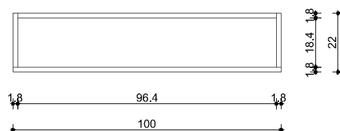
PRESJEK 1-1
