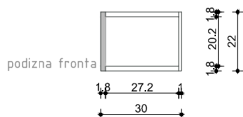
PRESJEK 2-2
