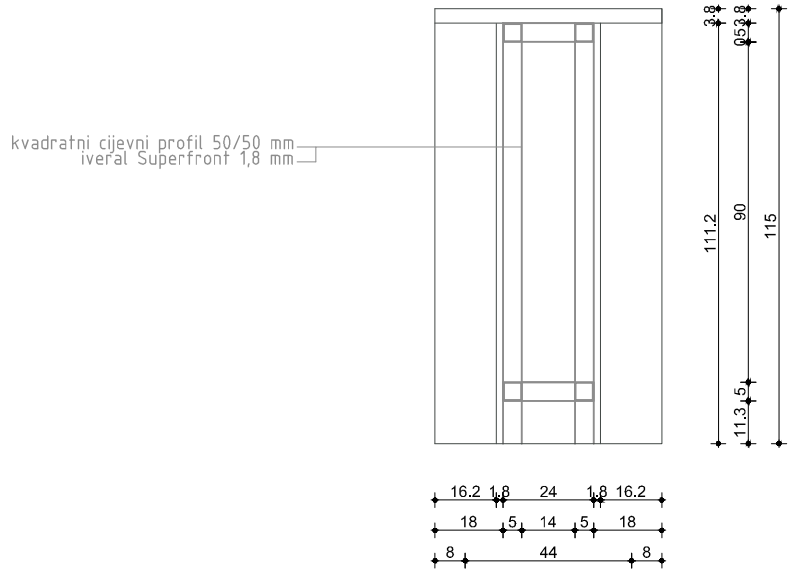
PRESJEK 2-2
