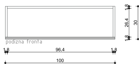
HORIZONTALNI PRESJEK
