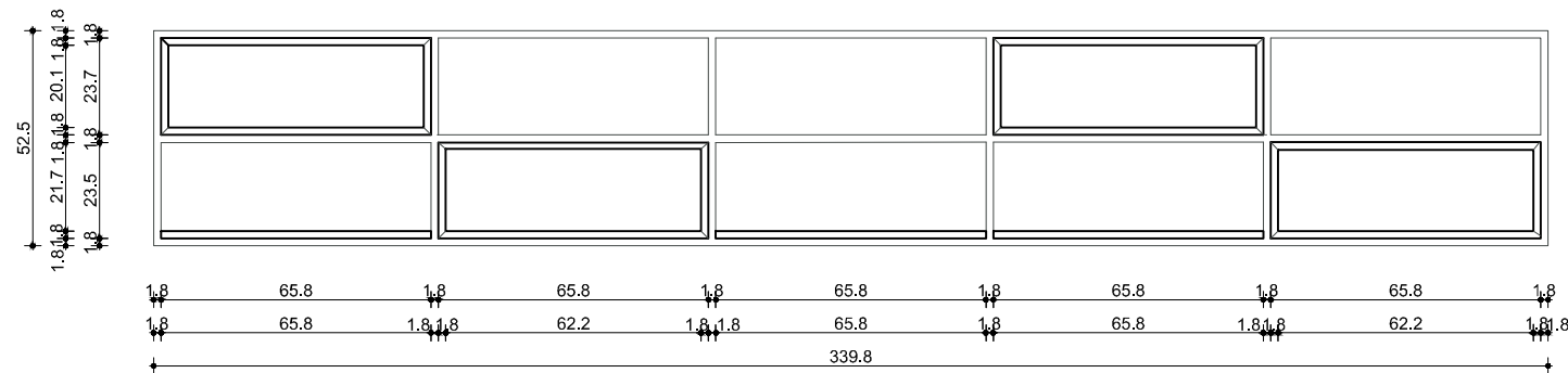
HORIZONTALNI PRESJEK
