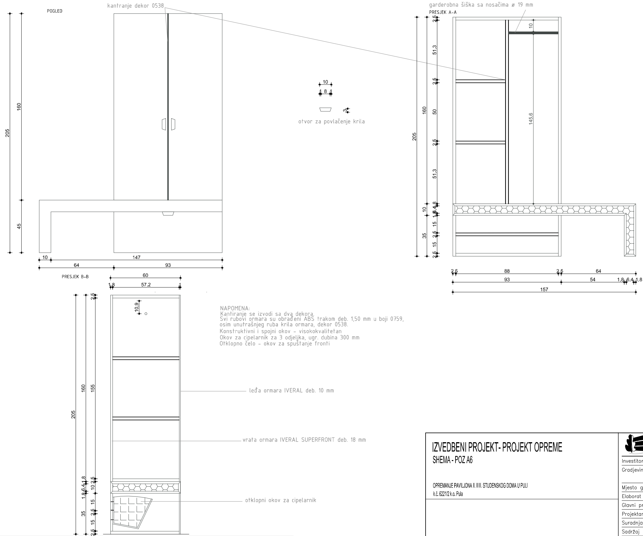
ZATVORENI GARDEROBNI ORMAR SA INTEGRIRANIM KLUPICOM
