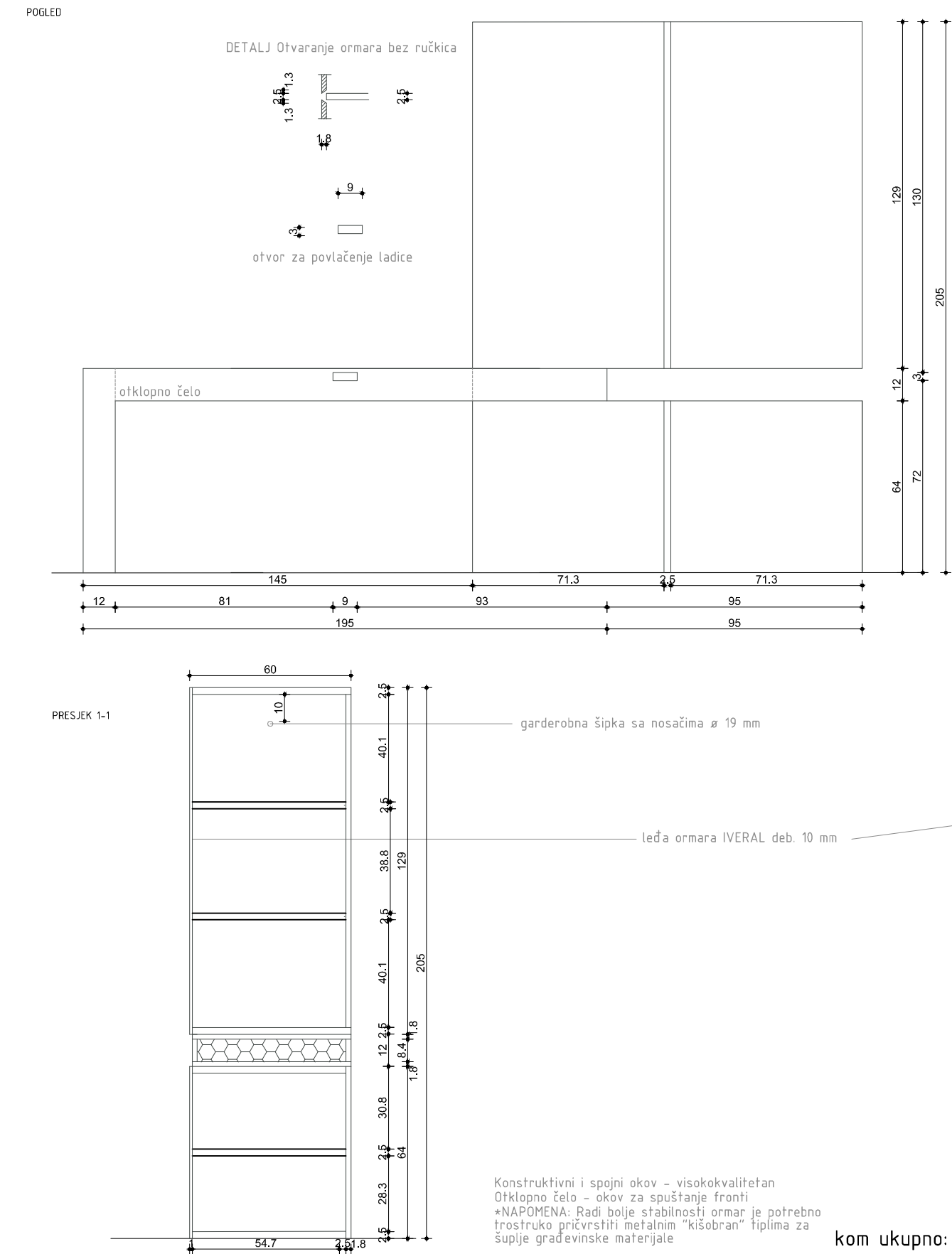
ZATVORENI GARDEROBNI ORMAR SA INTEGRIRANIM STOLOM
