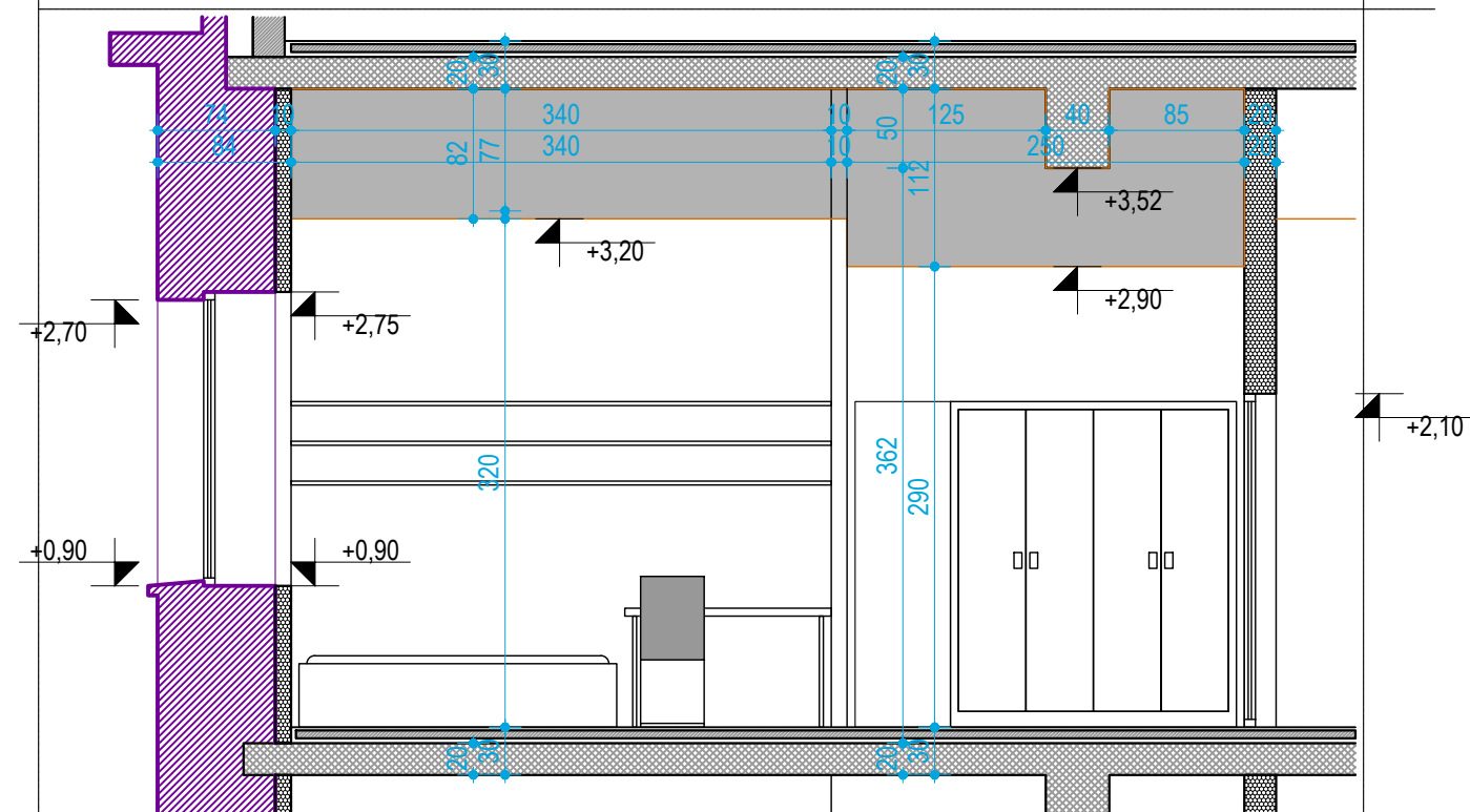
PRESJEK C-C
