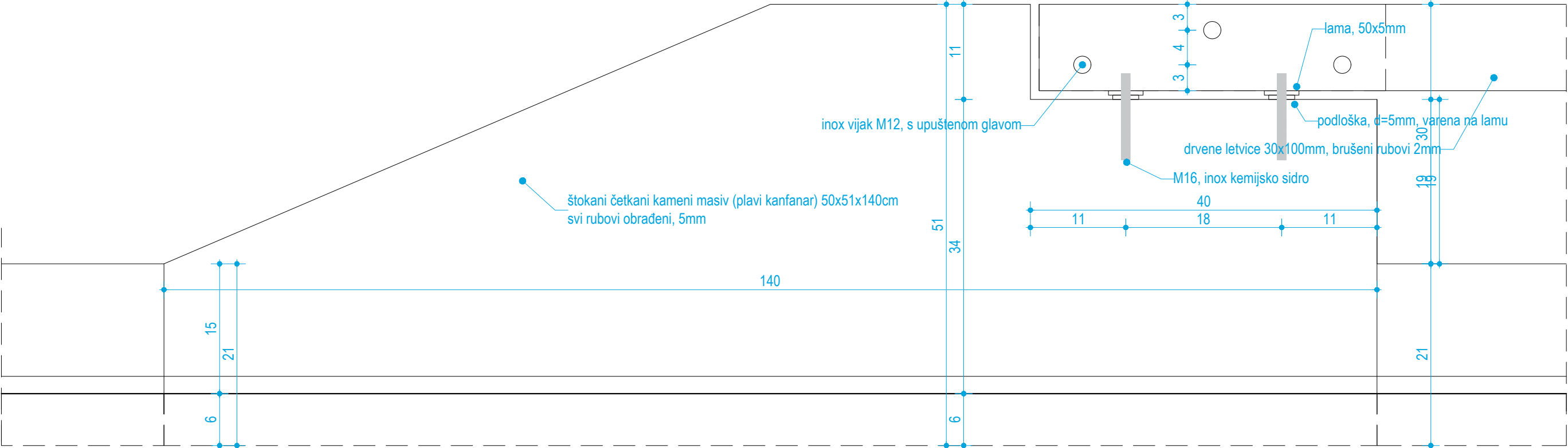
pogled, pozicija 1
