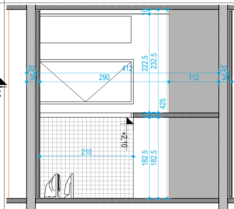
PRESJEK B-B
