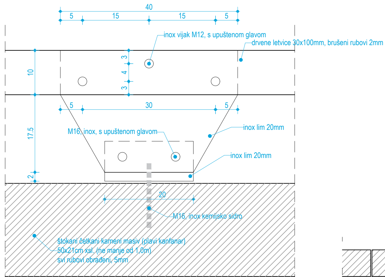
pogled, pozicija 2
