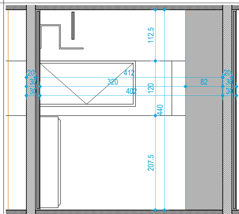
PRESJEK A-A
