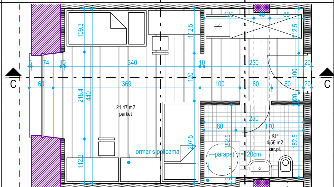
TLOCRT
